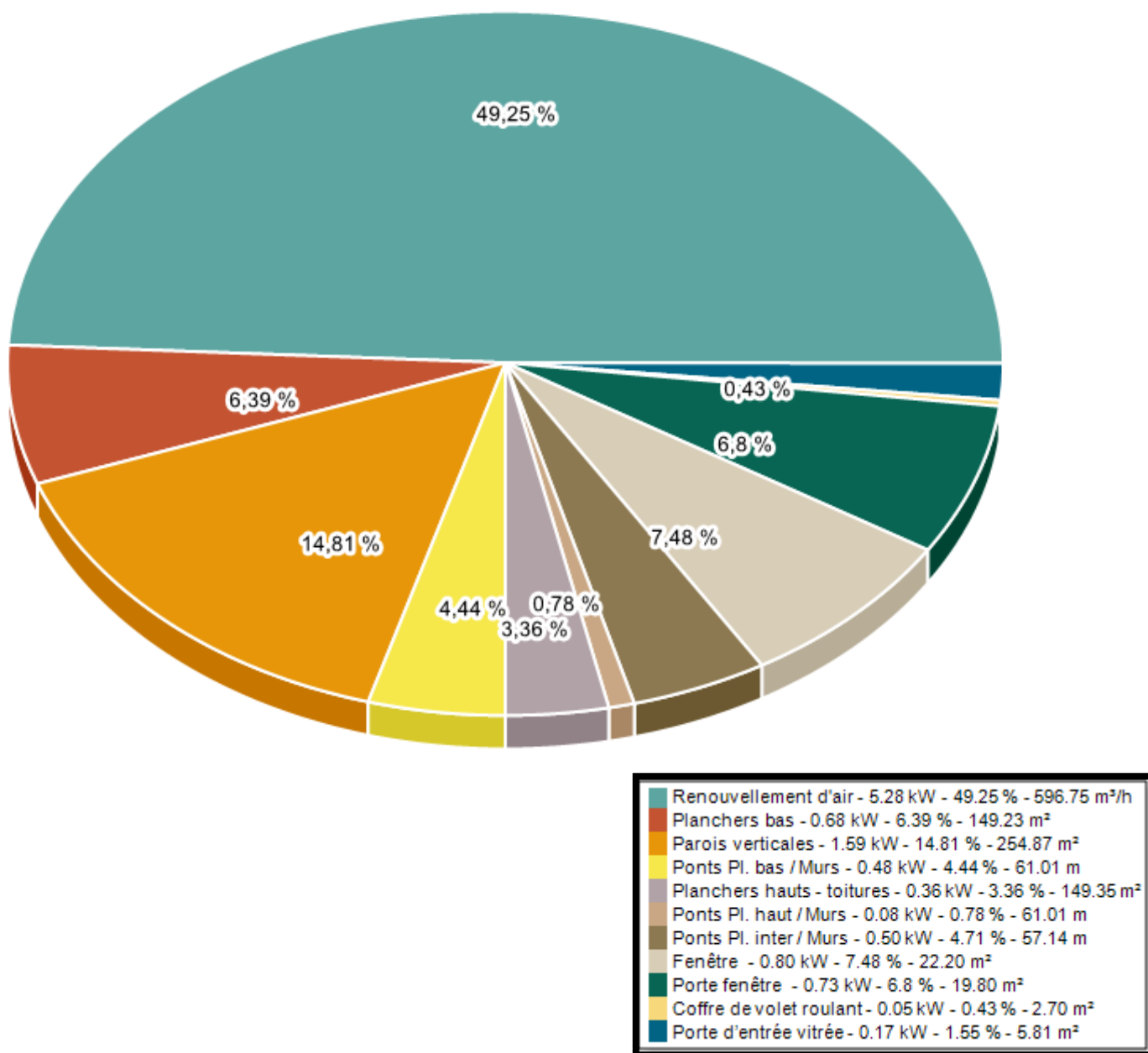
Répartition des déperditions poste par poste
